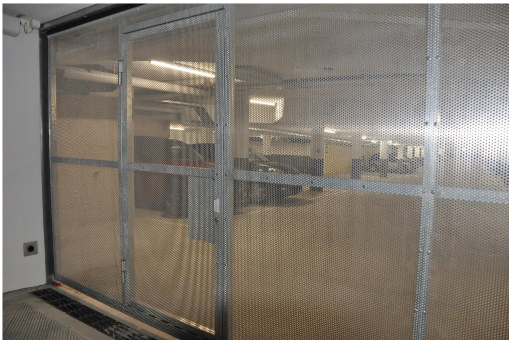
Sammelgaragen Schiebetor ST500 mit Schlupftüre Füllung Aluminium-Lochblech, Feuerverzinkt
